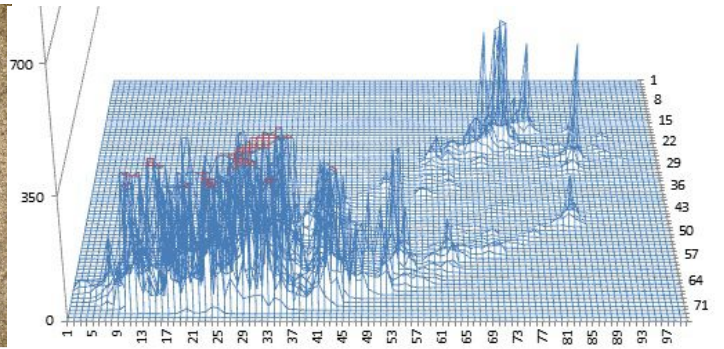
赤は荷重20gfで300Ω以上のポイント
