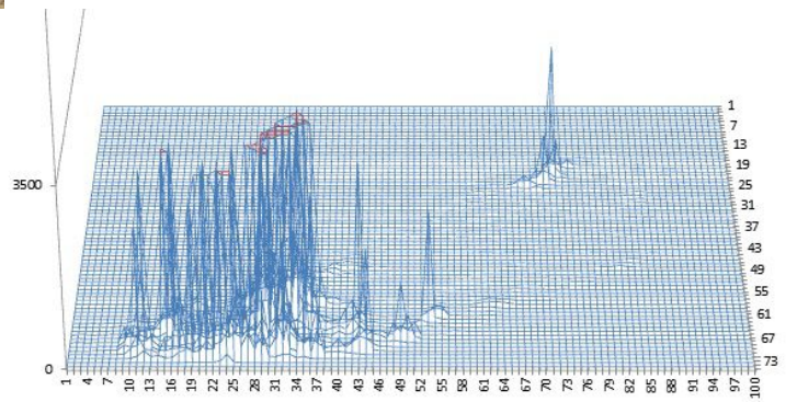
赤は荷重20gfで3.5KΩ以上のポイント
