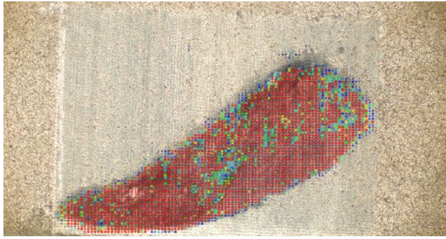
赤は荷重20gfで35Ω以上のポイント
