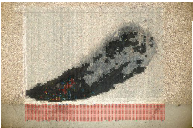
赤は荷重20gfで3.5KΩ以上のポイント
