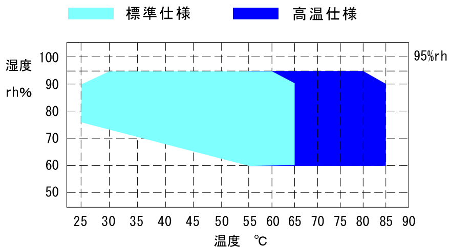
温湿度制御範囲図
